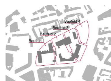
Bestand & Baufelder
